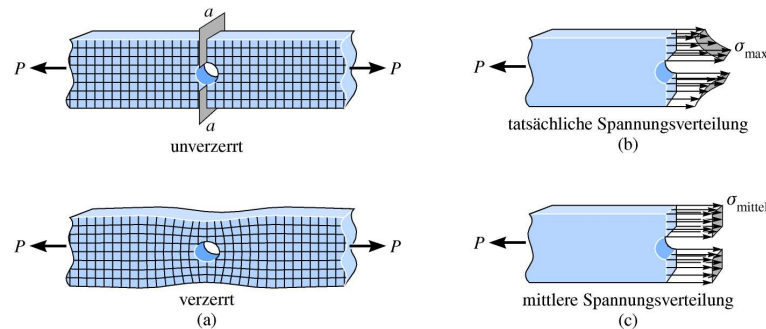
Abb.: Spannungskonzentration [1]
