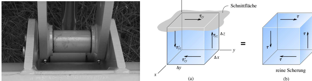
Abb.: Gelenkbolzen (links); Schubspannung (rechts) [1]
