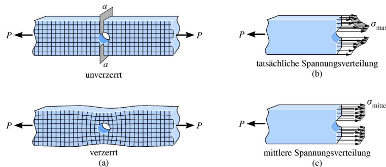
Abb.: Spannungskonzentration [1]
