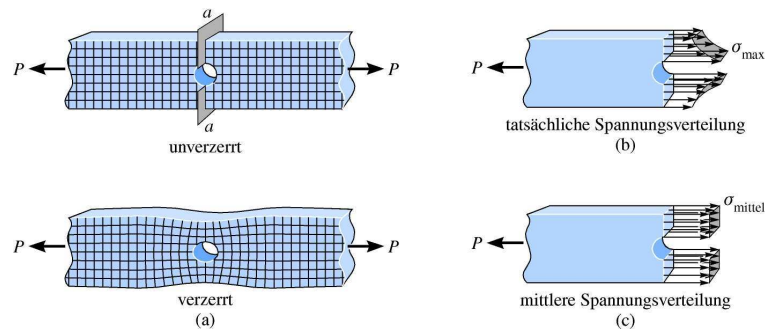
Abb.: Spannungskonzentration [1]
