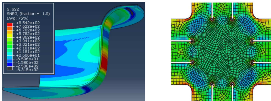
Simulation eines Tiefziehversuchs (links), FE-Modell einer Biaxialprobe (rechts)
