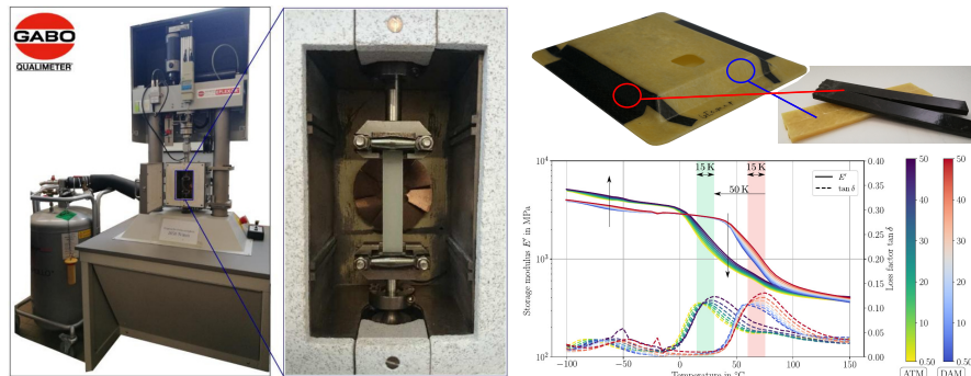
Abbildung 1: Dynamisch-mechanische Analyse mittels GABO Eplexor ® 500N (l.), Demonstratorbauteil und faserverstärkte Polymerproben aus dem GRK 2078 (r.o.), frequenz- und temperaturabhängige Materialantwort eines thermoplastischen Polymers (r.u.).
