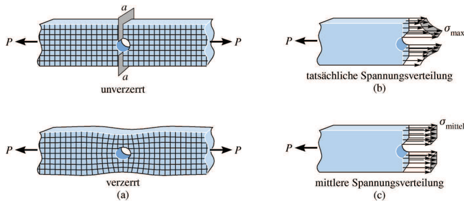
Abb.: Spannungskonzentration [1]
