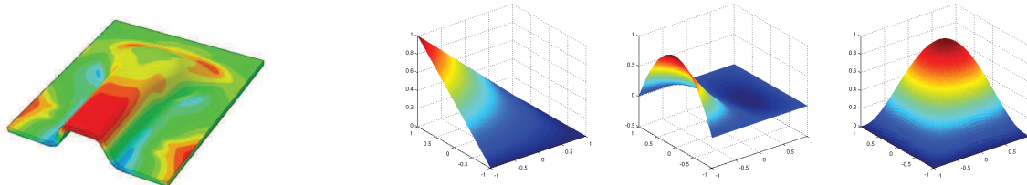
Abbildung: Lokale Spannungsanalyse eines langfaserverstärkten Polymers/Duromers im GRK 2078, www.grk2078.kit.edu (links); Bi-lineare und bi-quadratische Ansatzfunktionen (rechts)
